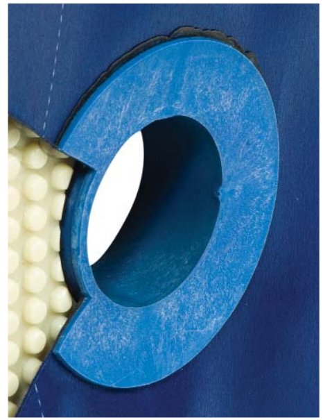
Cuello de alimentación de HPR soldado, patentado por Micronics
